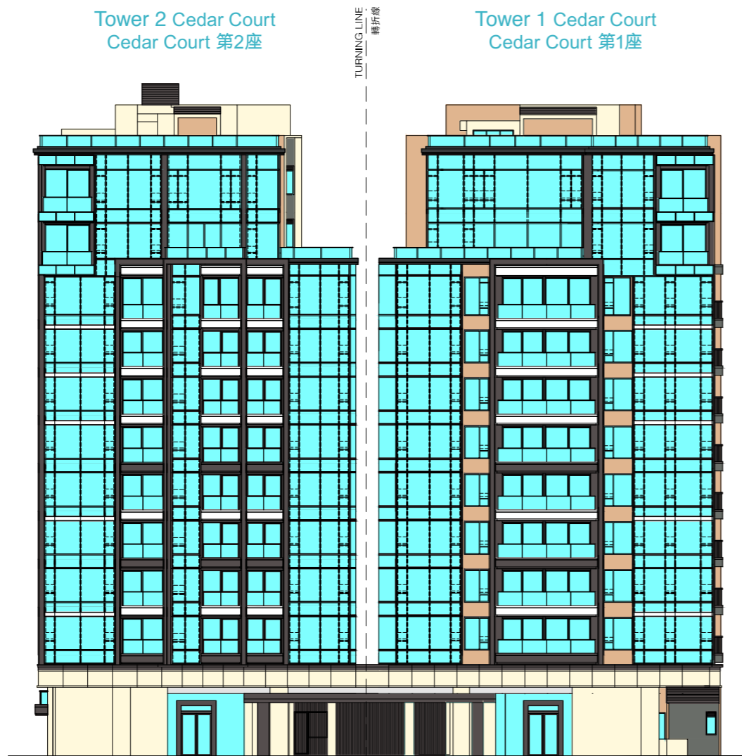
Elevation Plan B3 立面圖 B3
