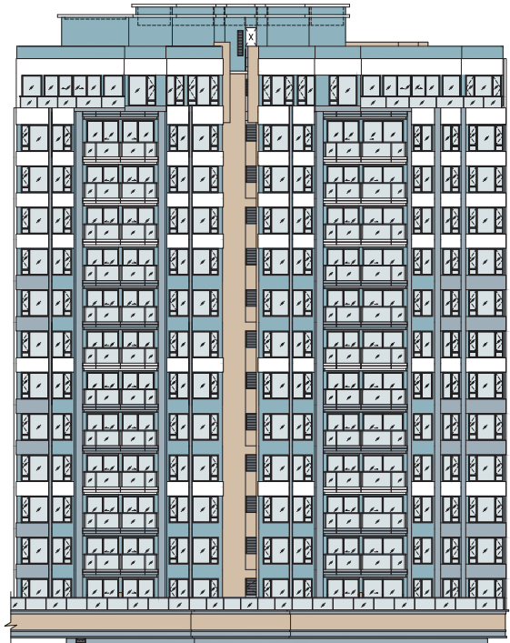
Elevation 4 立面 4
