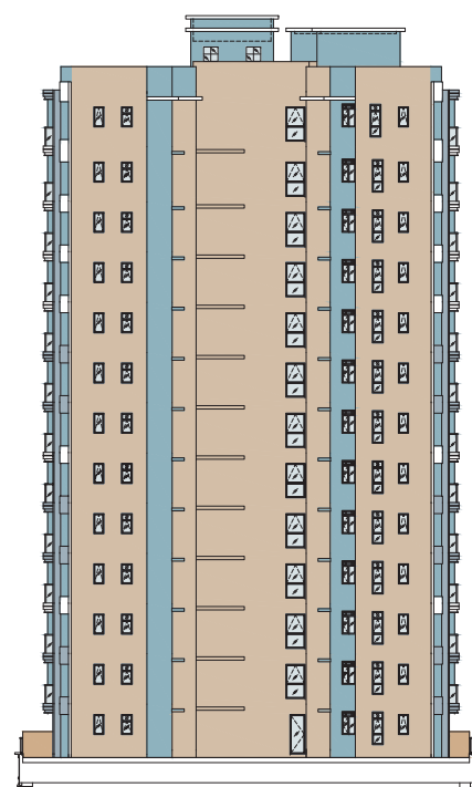
Elevation 3 立面 3
