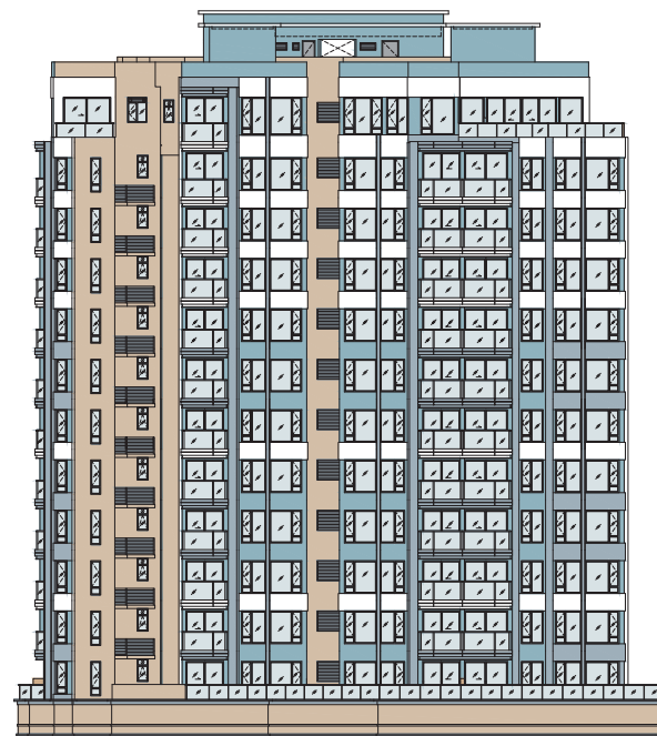
Elevation 2 立面 2
