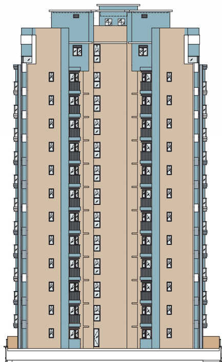
Elevation 1 立面 1
