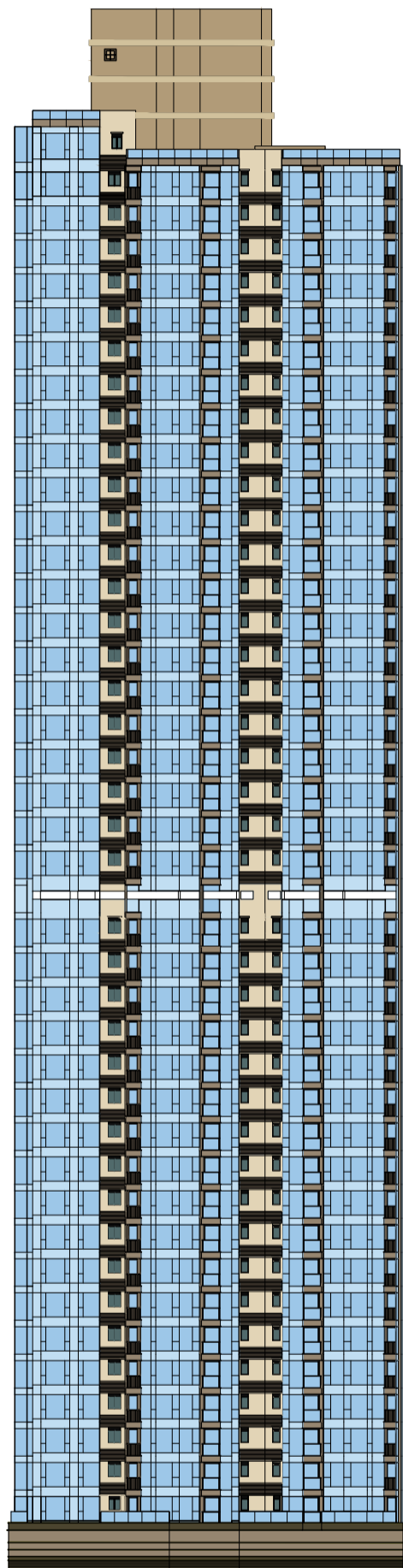
ELEVATION 1 立面圖 1
