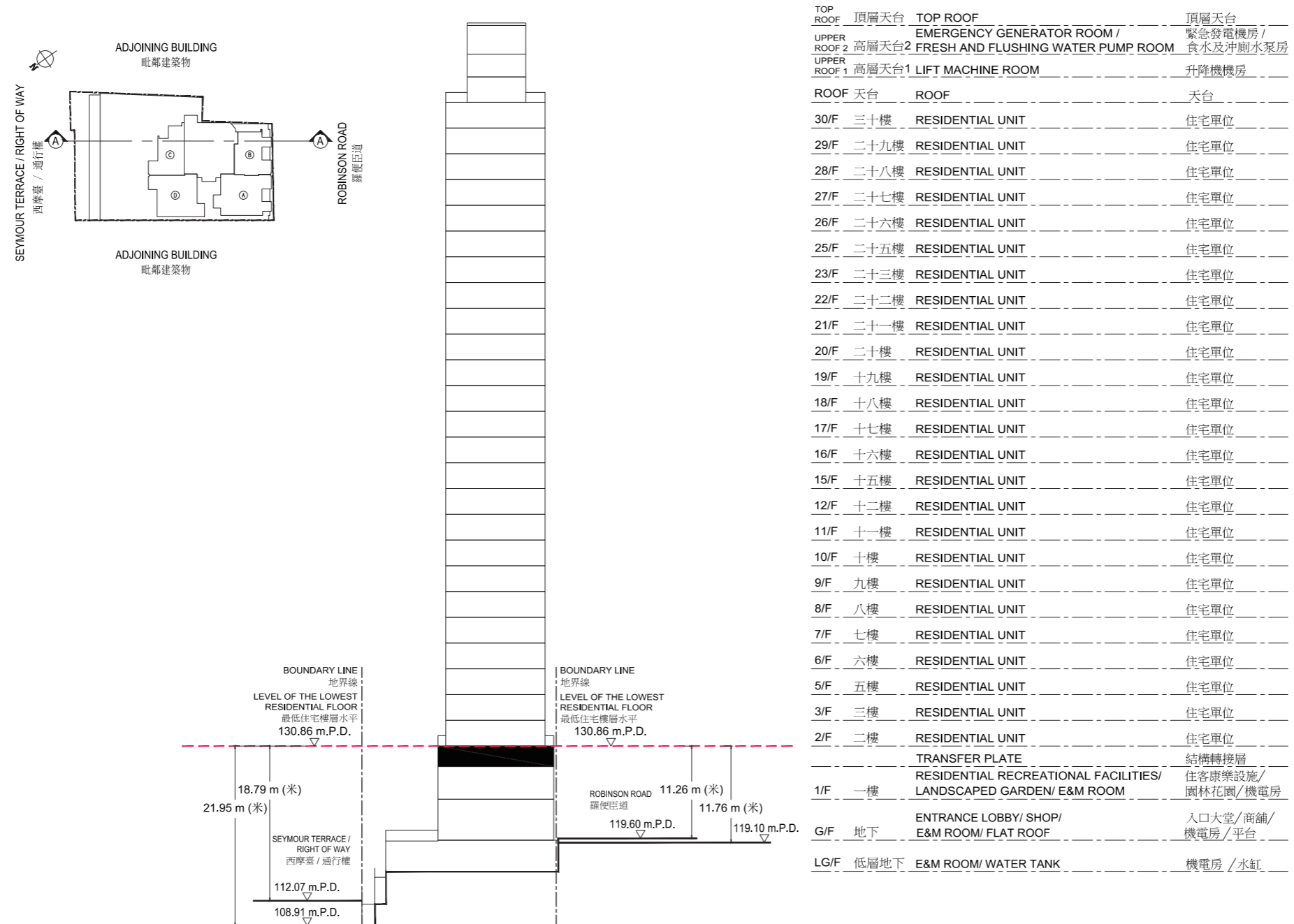
橫截面圖 A-A CROSS-SECTION A-A
