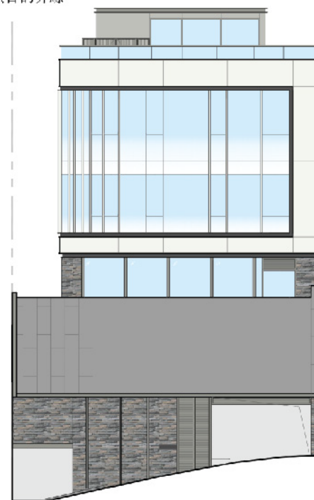
ELEVATION PLAN E2 立面圖 E2
